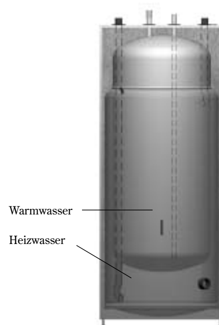
Doppelwandiger Warmwasserbereiter
